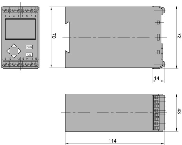
Bild 10: Einbauzeichnung
